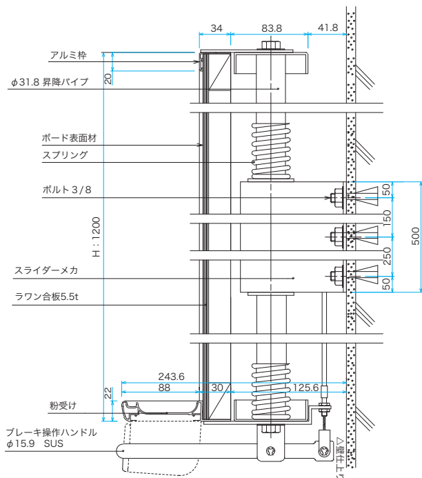
縦断面図
