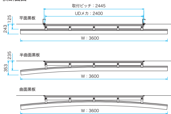
横断面図
