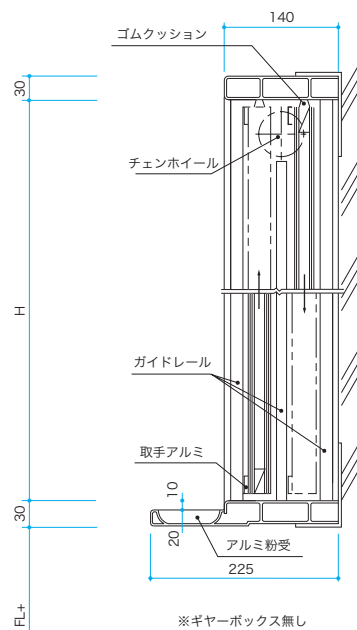
縦断面図
