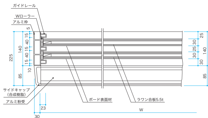
横断面図
