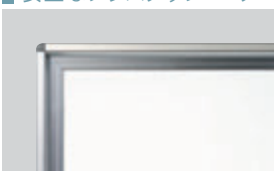
MH36TDYN ¥92,200 外形寸法 / W1926×D610×H1840 板面寸法 / W1810×H910 有効寸法 / W1770×H870
