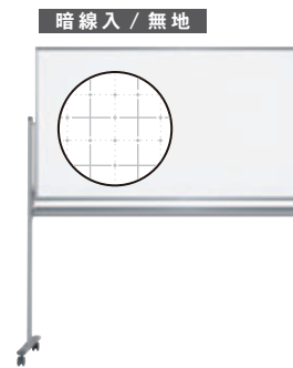
MH36TDXN ¥93,500 外形寸法 / W1926×D610×H1840 板面寸法 / W1810×H910 有効寸法 / W1770×H870
