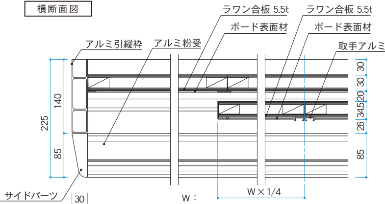
横断面図
