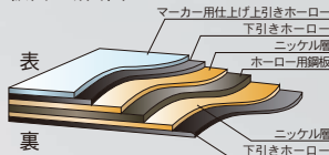
板面 断面図
