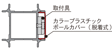
ポール断面図
