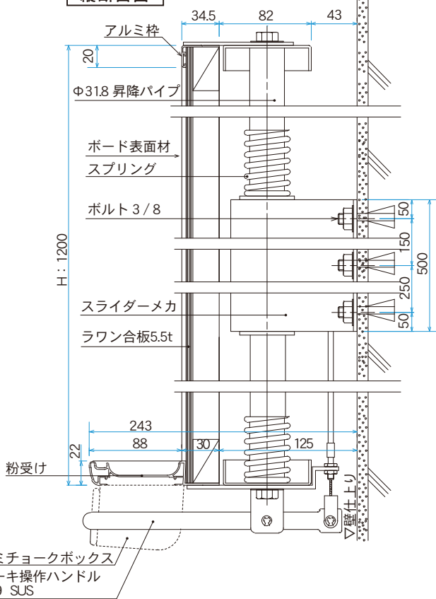
縦断面図
