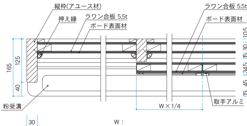
横断面図
