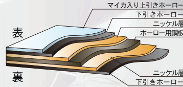
板面 断面図
